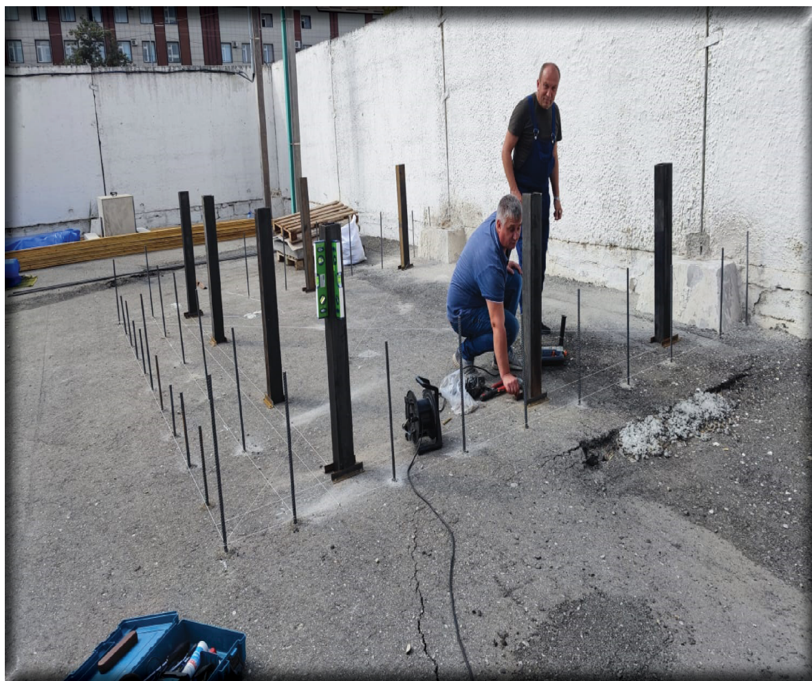
Возведение основания
